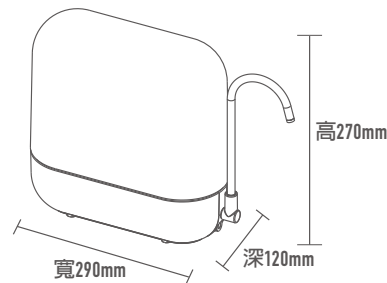
UP-602PP 潔淨組尺寸
