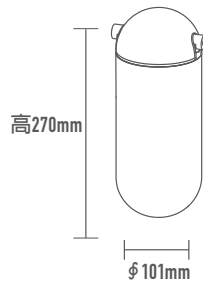
UP-601 單道淨化組尺寸
